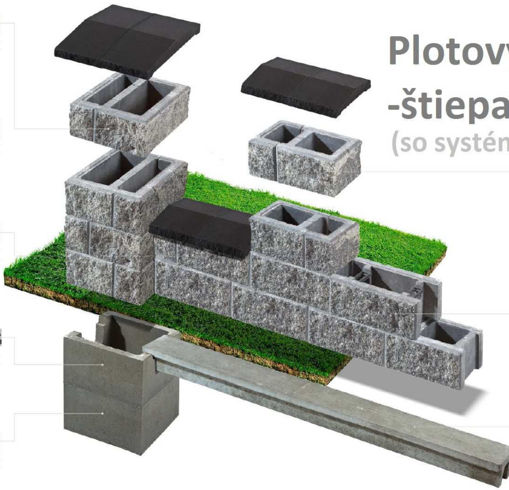
BLOK STĽPOVÝ (+ukončovaci pre múr hr.38) symbol: B2 váha: ok. 25,5 kg
