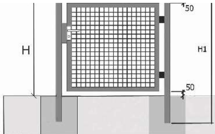
Bránka jednokrídlová s rebierkovou výplňou Alt.2
