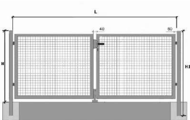
Bránka dvojkřídlová s rebierkovým pletivom. Alt.2
