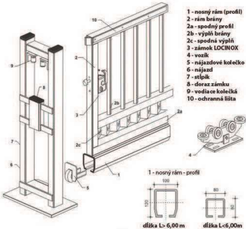
Detail - brána samonosna, typ BST
