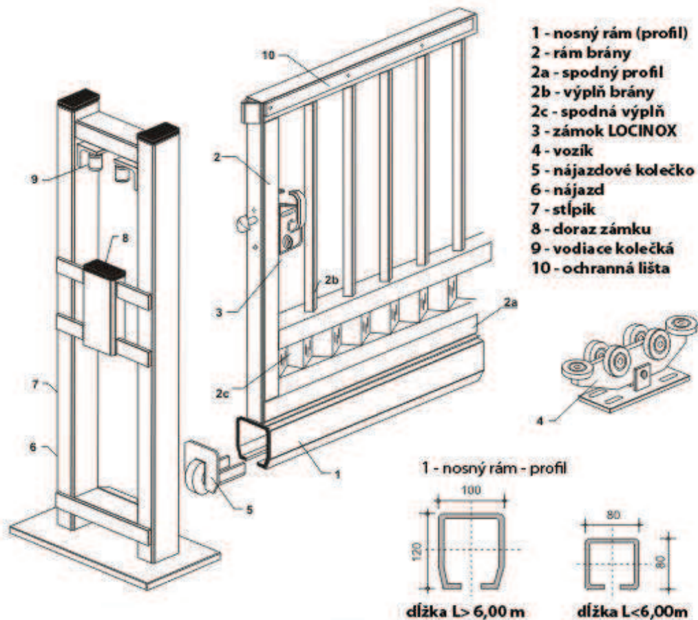
Detail - brána samonosna, typ BST
