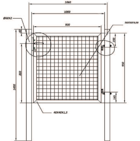
Bránka ECO 1000 x 1000
