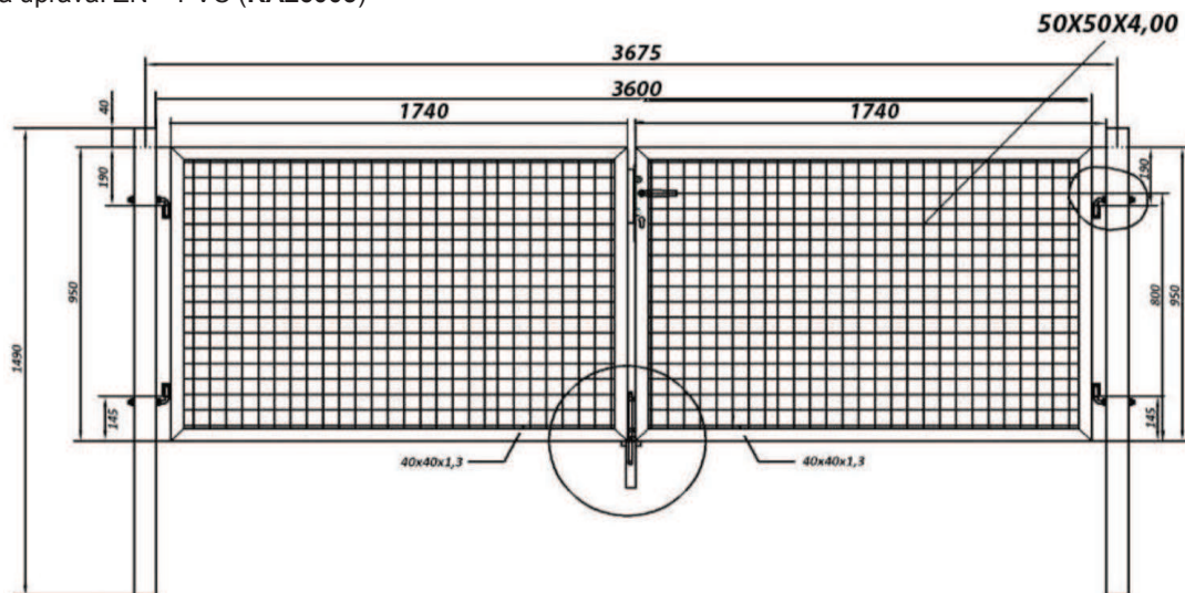
BRÁNA ECO 1000 X 3600
